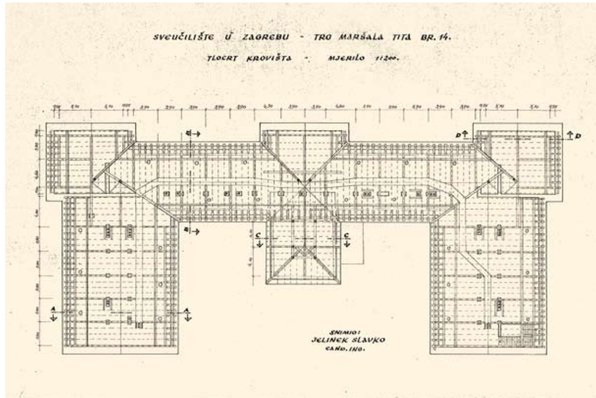
84. Tlocrt krovišta, snimak stanja oko 1949.
