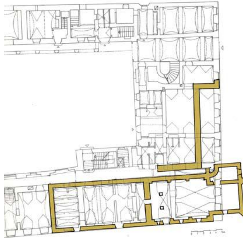
1. Hospital i kapela B. D. Marije na Gradecu u 17. stoljeću ucrtani na tlocrtu jugoistočnog dijela razizemlja Banskih dvora Nacrt: Mladen Perušić
