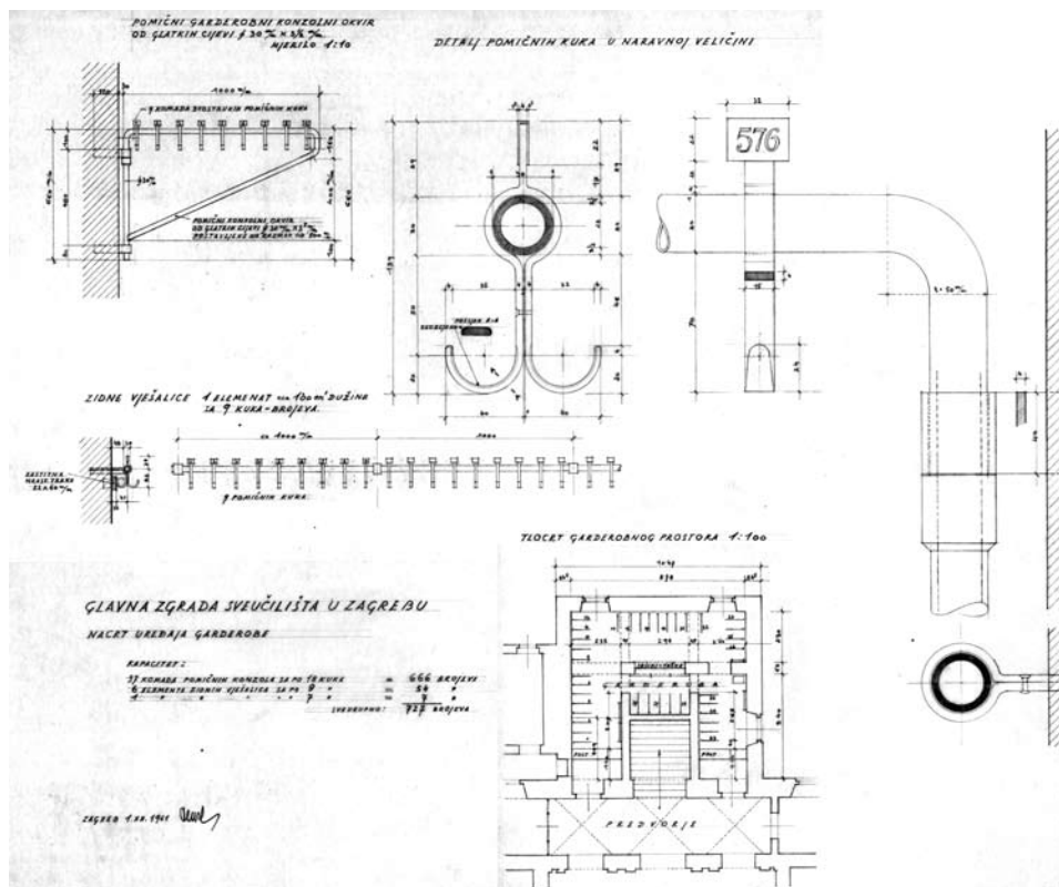
1. Projekt garderobe u prizemlju iz 1961.
