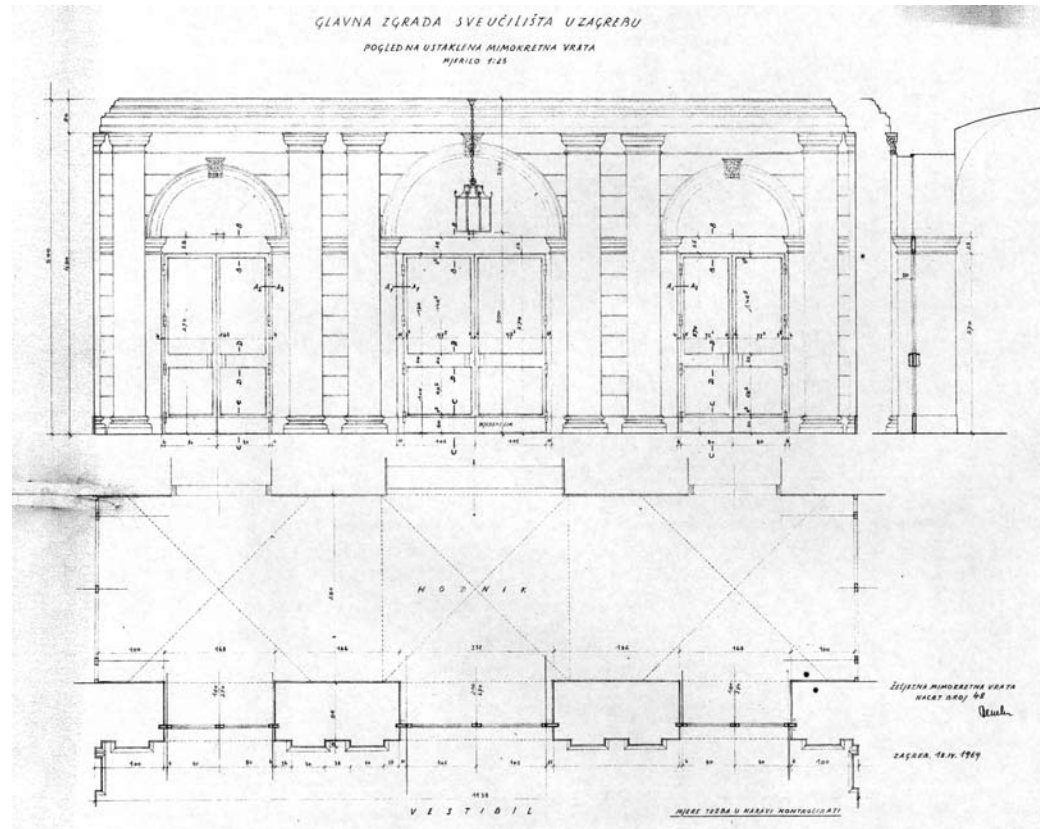
34. Nacrt mimokretnih vrata vestibula, 1969.
