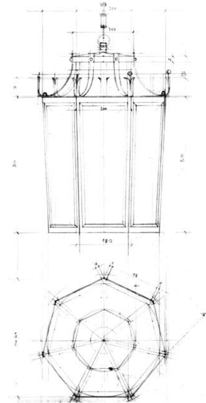
12. Viseća svjetiljka u vestibulu – detalj nacrtu
