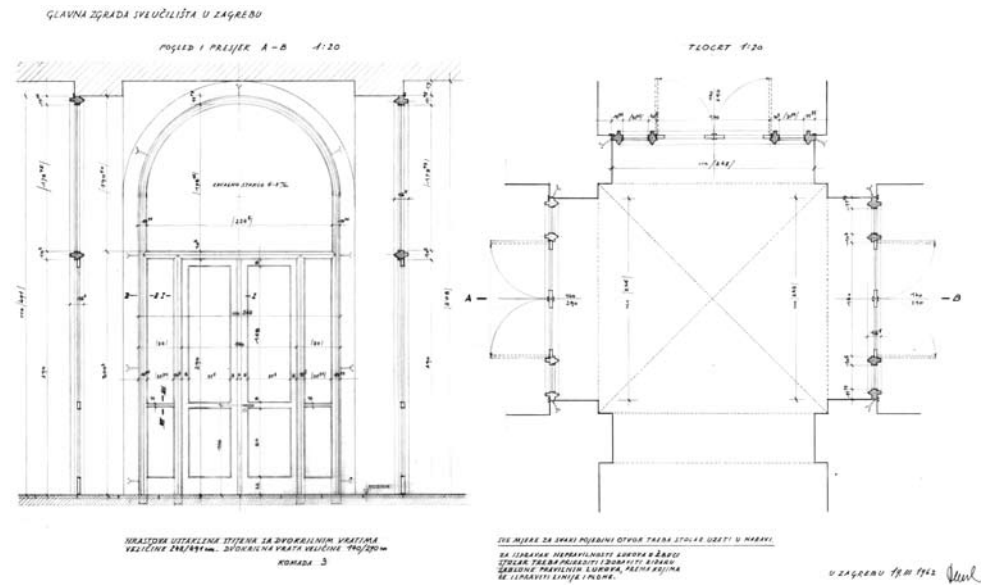
6. Nacrt drvene ostakljene stijene
