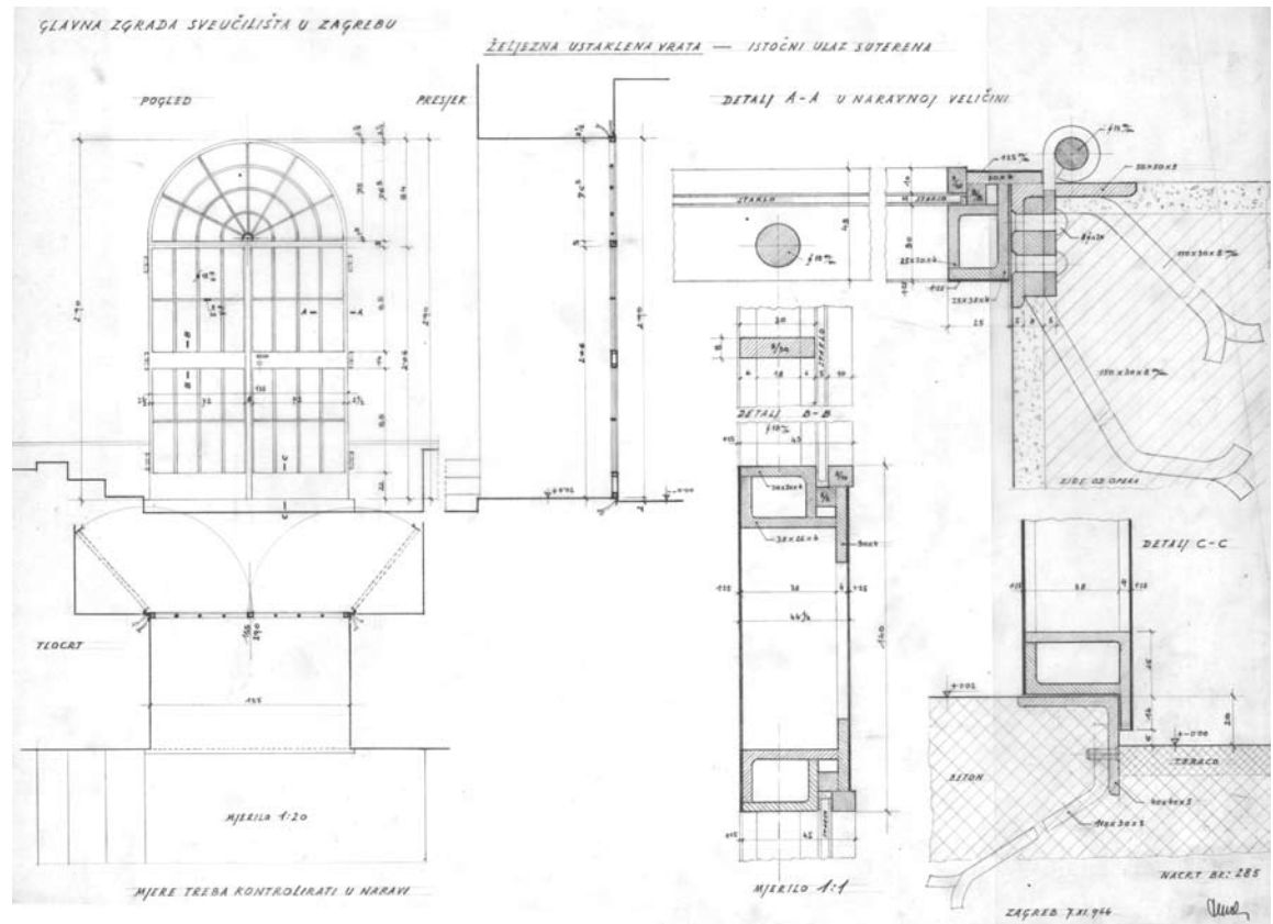
20. Projekt suterenskih vrata južnog pročelja
