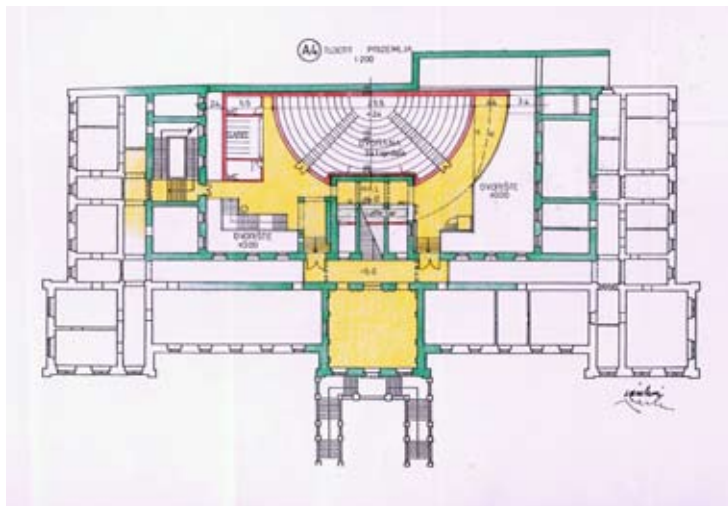
M. Čanković i I. Juras: Tlocrt dogradnje dvorane u dvorištu zgrade Sveučilišta, 2002.
