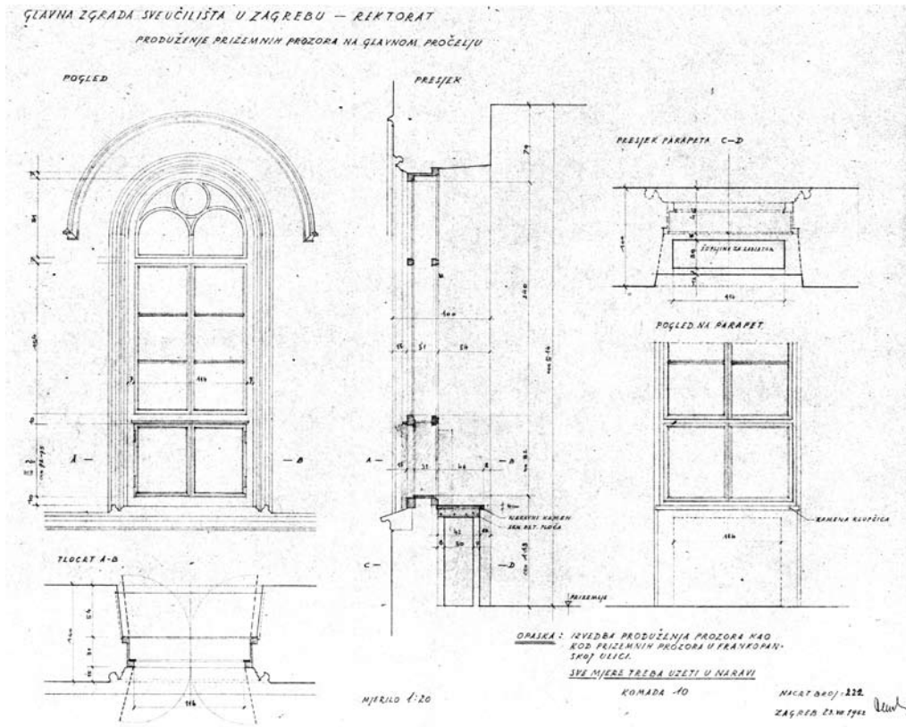
4. Projekt produljenja prozora prizemlja na južnom pročelju
