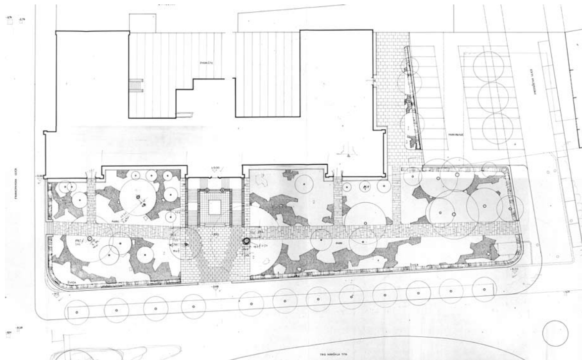
Juraj Denzler: Plan uređenja Sveučilišnog perivoja, 1966.
