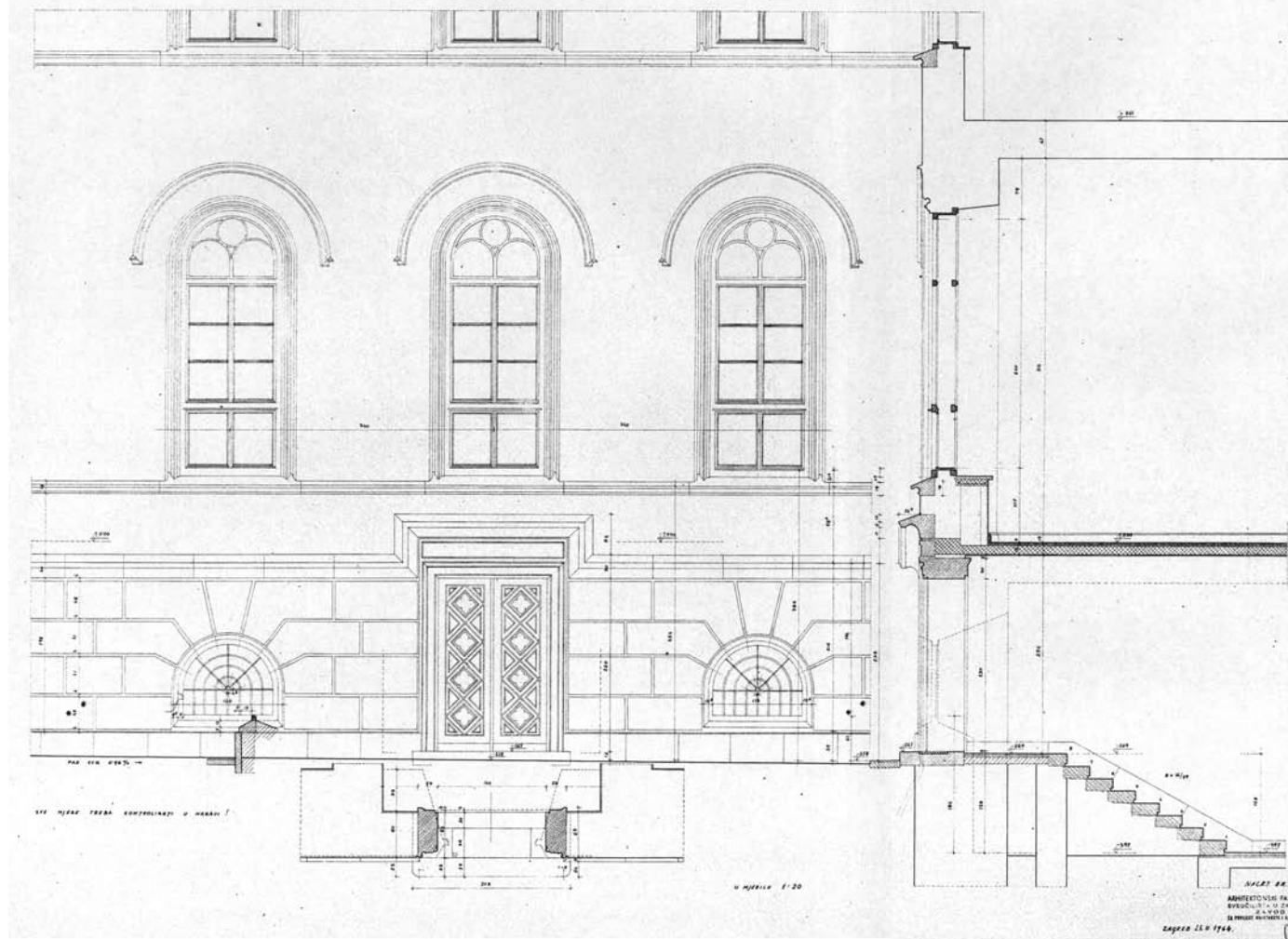
7. Denzlerov projekt za ulazni portal u Frankopanskoj ulici
