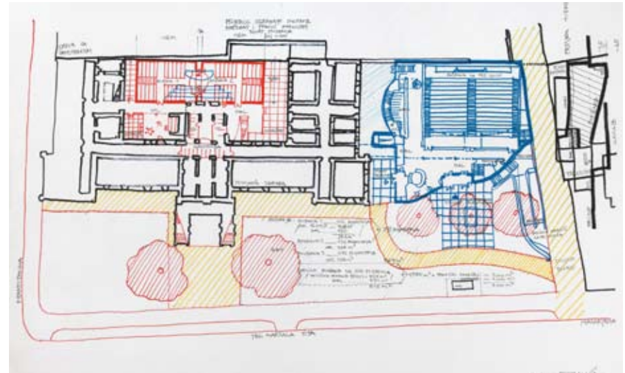
M. Čanković i I. Juras: Tlocrt dogradnje Pravnog fakulteta, 1998.
