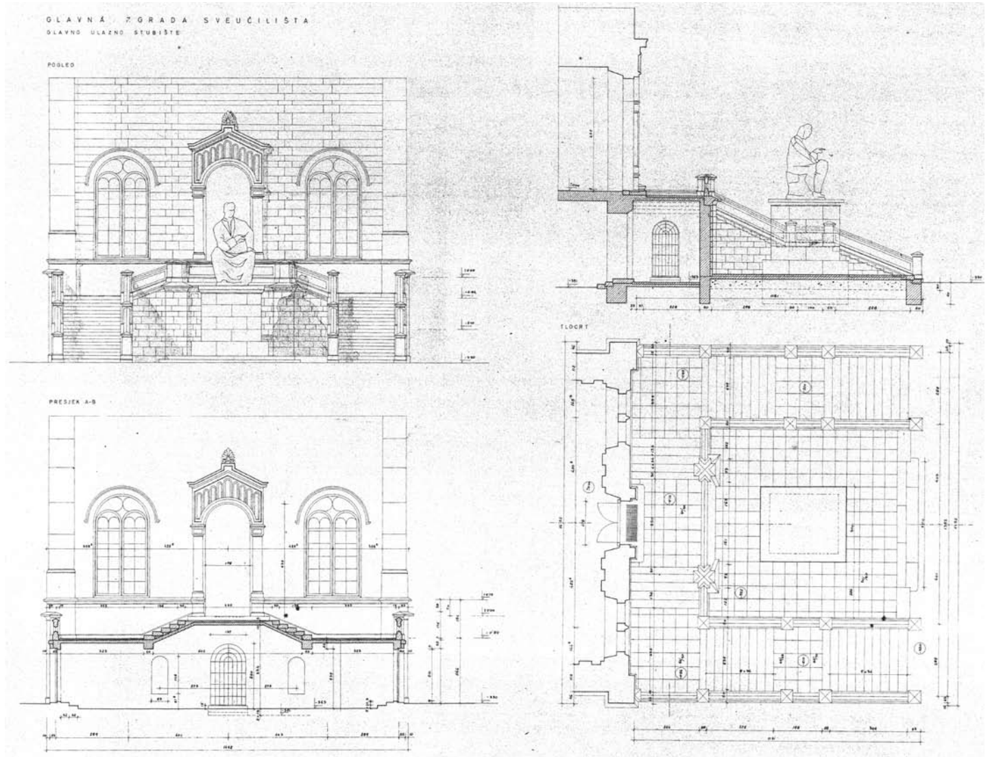
8. Projekt obnove ulaznog stubišta 1963.
