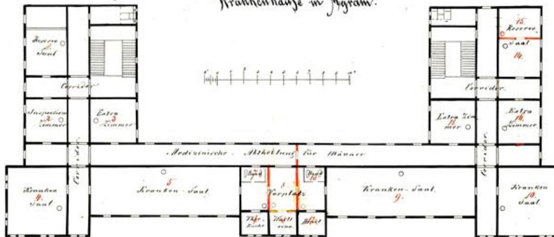
Grundriss Skizze des Erdgeschosses vom allgemeinen Krankenhaus in Agram.
