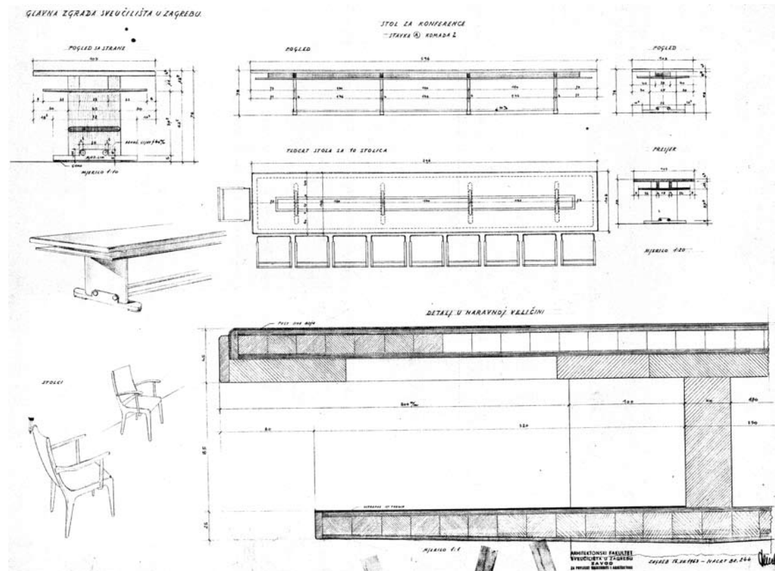
4. Izvedbeni nacrt stola za konferencije
