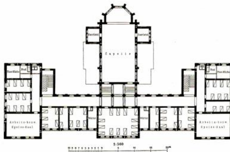
3. Gradska bolnica u Berlinu 1889., arh. Blankenstein
